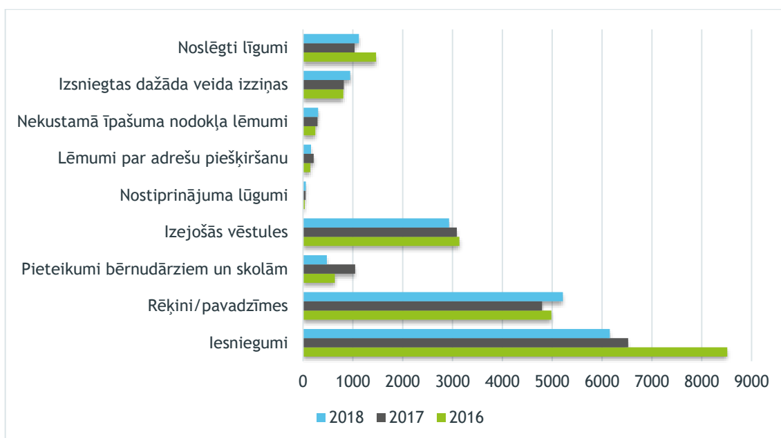
6. attēls. Ķekavas novada VPVKAC veiktie pašvaldības pakalpojumu dinamika 2016.- 2018. gadā
